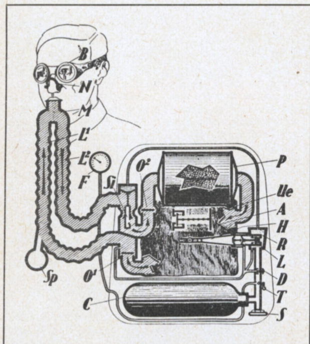
Schematische Darstellung eines Sauerstoff-Kreislaufgerätes, dessen Bau- und Wirkungsweise in unserem Artikel ausführlich geschildert werden.
