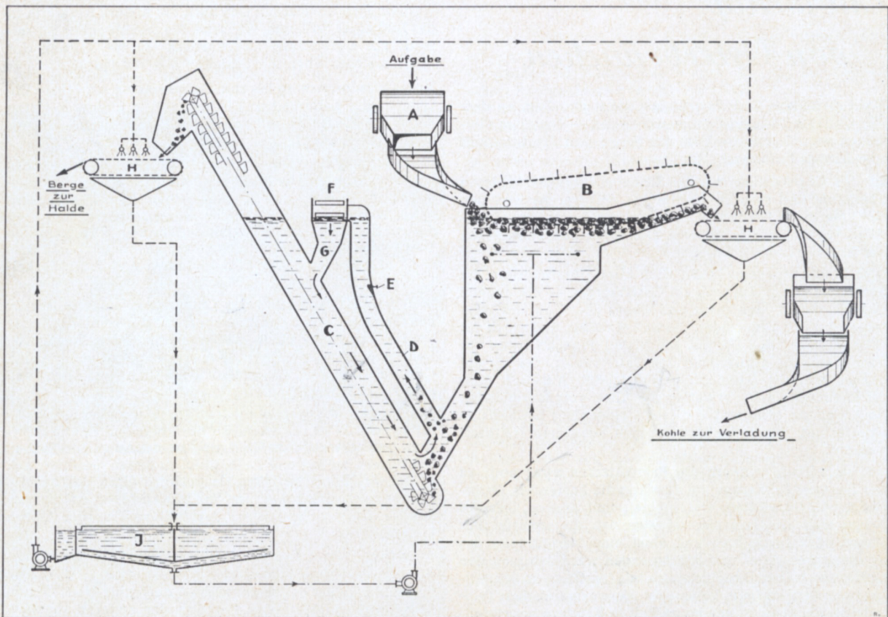
Schema eines Schwimmkastens
